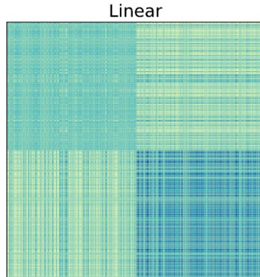
(a) PCA
