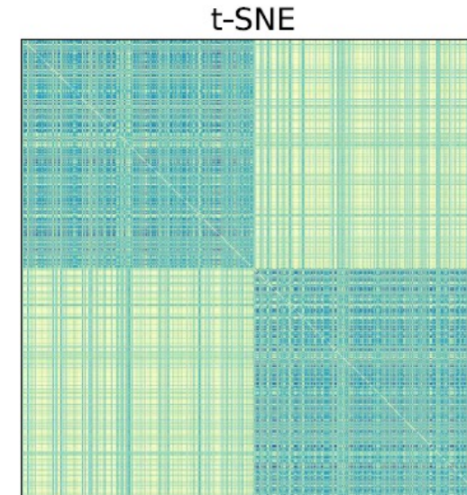
t-SNE
